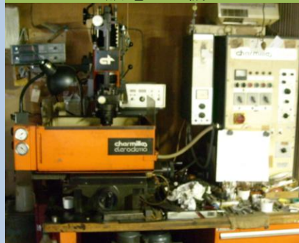
放電加工機
