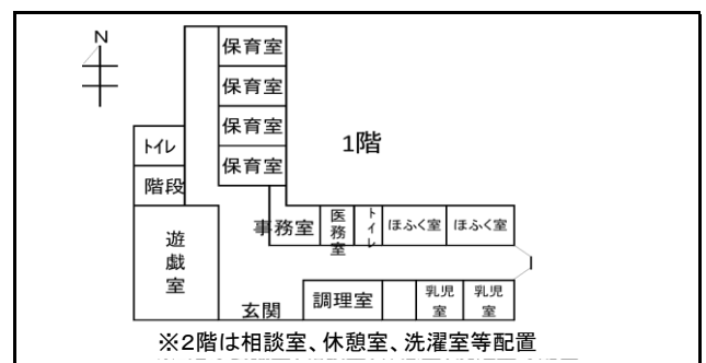
施設平面図
